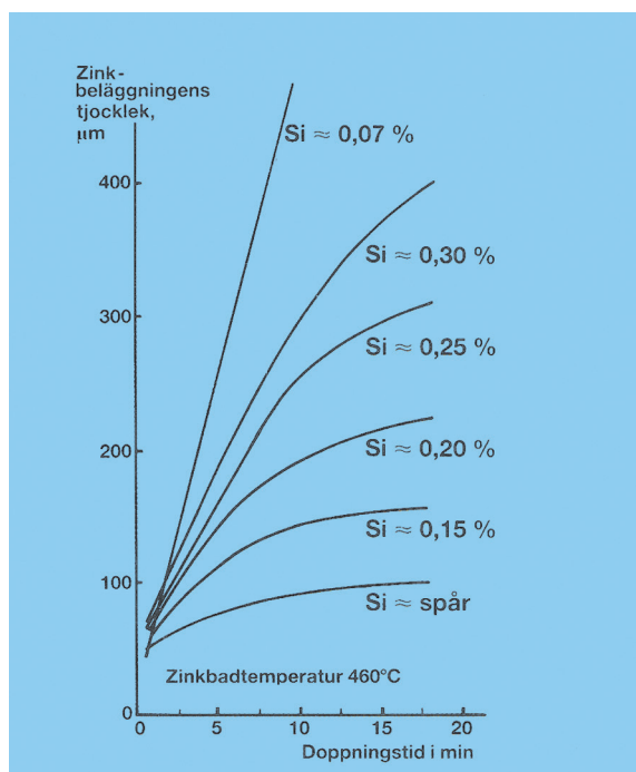
Figur 1. Förhållandet mellan dopptid och skiktthjocklek för stål med olika kiselhalter. Kurvorna är medelkurvor baserade på både studier och praktisk erfarenhet. Betydande variationer kan förekomma mellan stål med samma kiselhalt men från olika charger. Kurvorna gäller för ett zinkbad utan tillsats av nickel.
