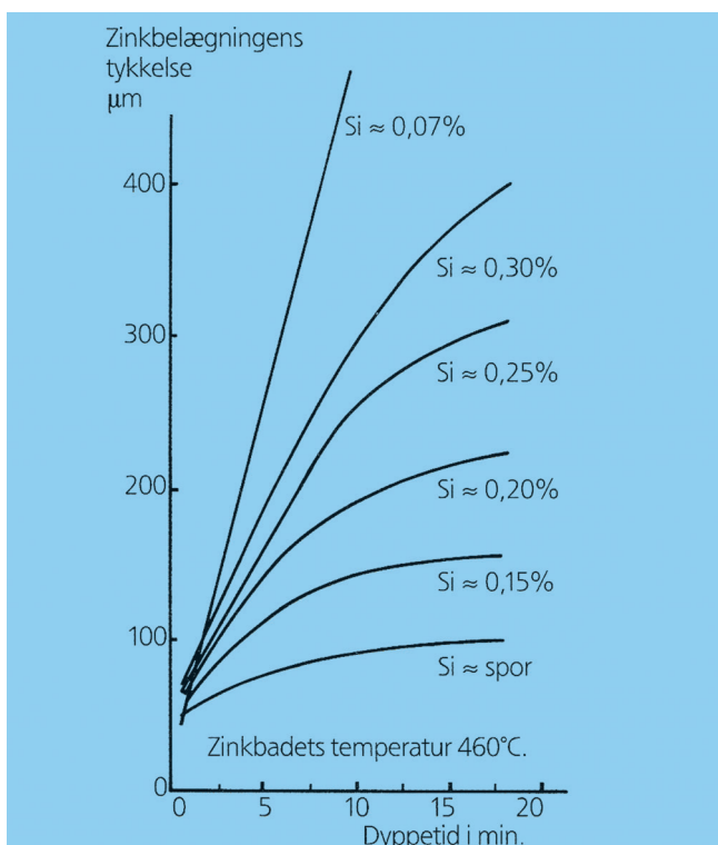
Figur 1. Forholdet mellem dyppetid og zinklagets tykkelse for stål med forskelligt siliciumindhold. Kurverne er middelmåder baseret på såvel undersøgelser som praktiske erfaringer. Der kan forekomme betydelige variationer mellem stål med samme siliciumindhold men fra forskellige charger. Kurverne gælder for et zinkbad uden nikkeltilsætning.
