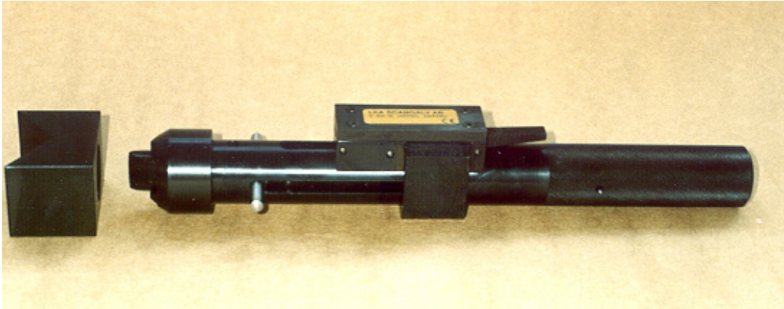
Slagmejsel för vidhäftningsprovning.
