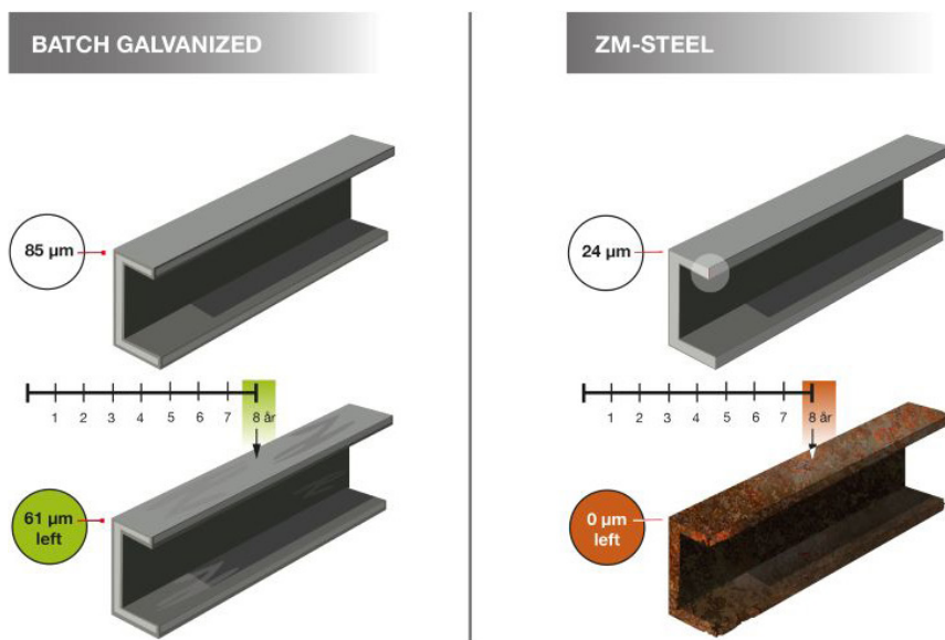
Figur 6. Studien visade att korrosionshastigheten för det styckvis förzinkade stålet och ZM-stålet var densamma efter ett par års exponering, och det som blir avgörande livslängden är skiktjockleken.
